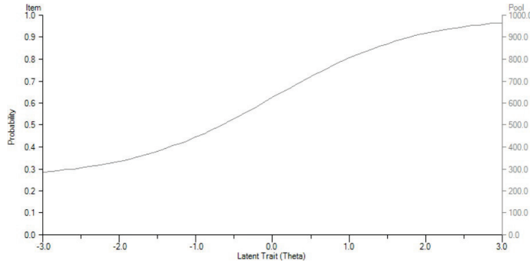
Şekil 1. Madde Havuzuna İlişkin Yanıt Fonksiyonu
